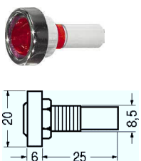
Signalna lučka z matico, brez kabla
