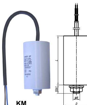
KM kabel +(matica) vijak M8
