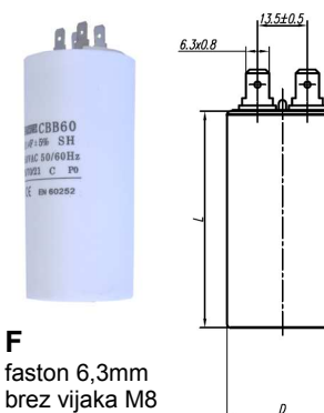
K kabel brez vijaka M8
